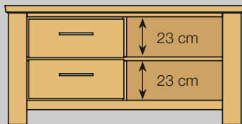
0204- Medienanrichte B 130 H 64 T 46 cm 2 Schubkästen, 2 offene Fächer lichtetes Maß der offenen Fächer: B 53 H 47 T 39 cm
