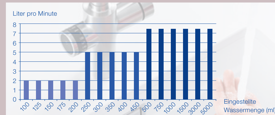
Dynamic Flow Control: Je mehr Wasser Sie brauchen, desto schneller fließt es durch die Leitung. Und Sie sind schneller fertig.
